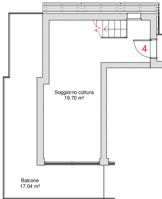
PIANO PRIMO
