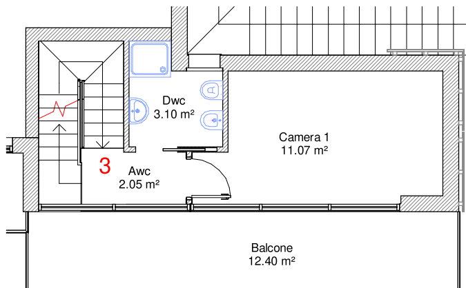
PIANO PRIMO
