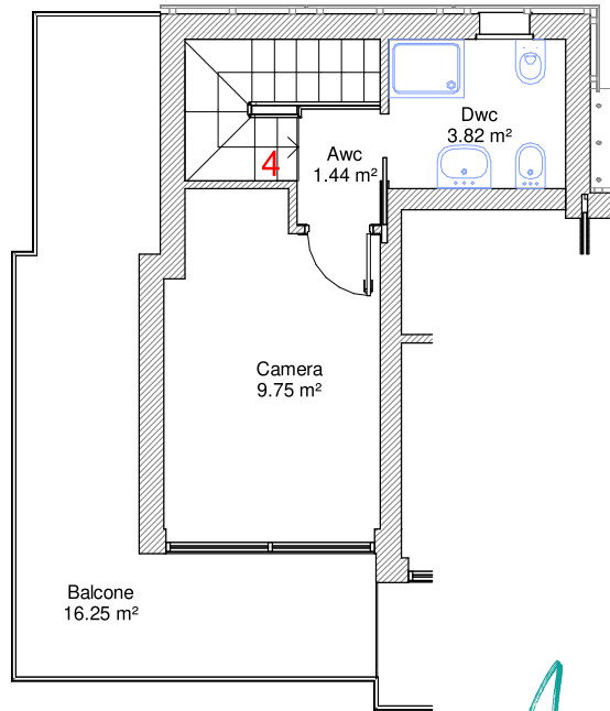
PIANO SECONDO
