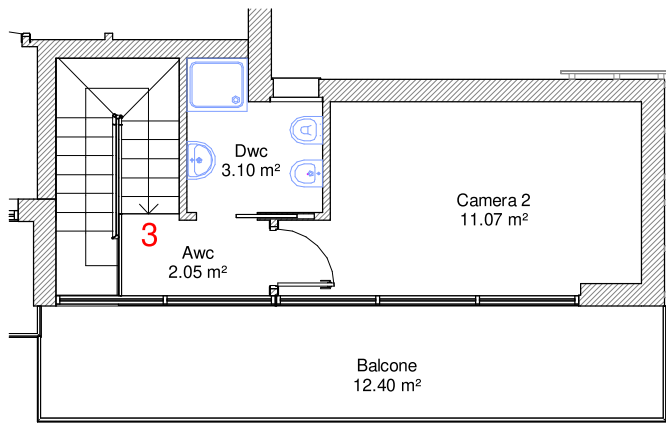
PIANO SECONDO
